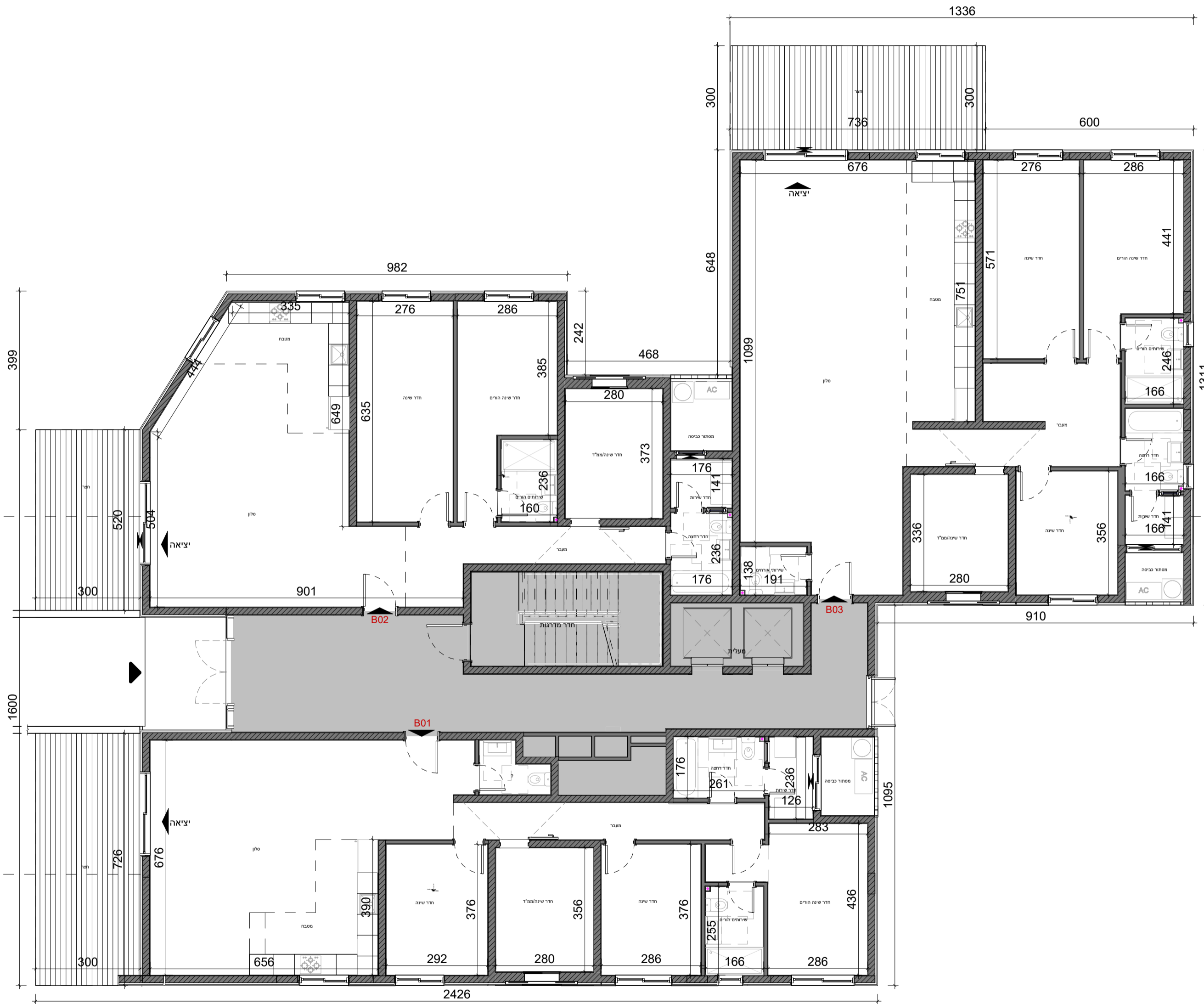
תכנית קומת קרקע 1:100 קנ"מ
