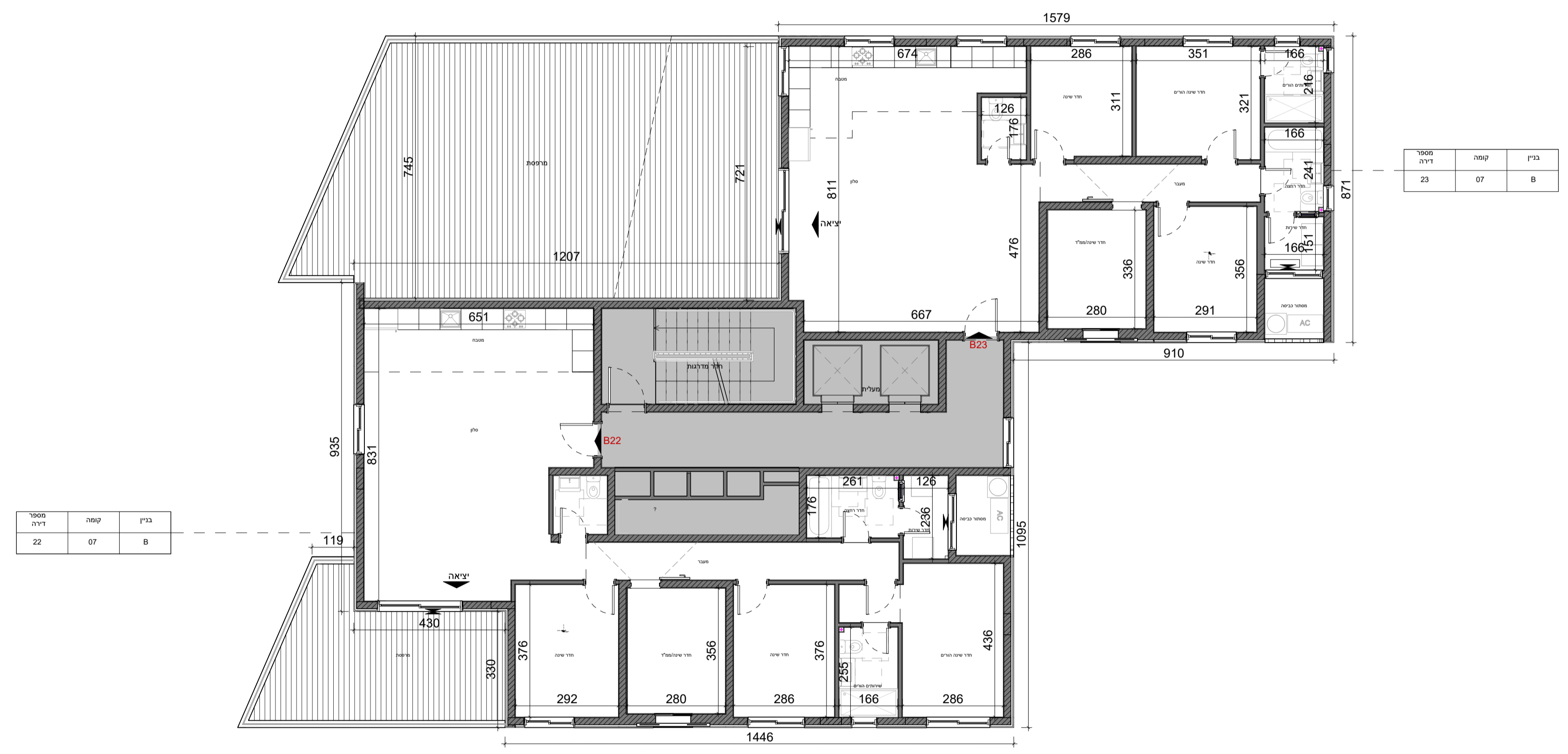
תכנית קומה שביעית 100 : 1 קנ"מ
