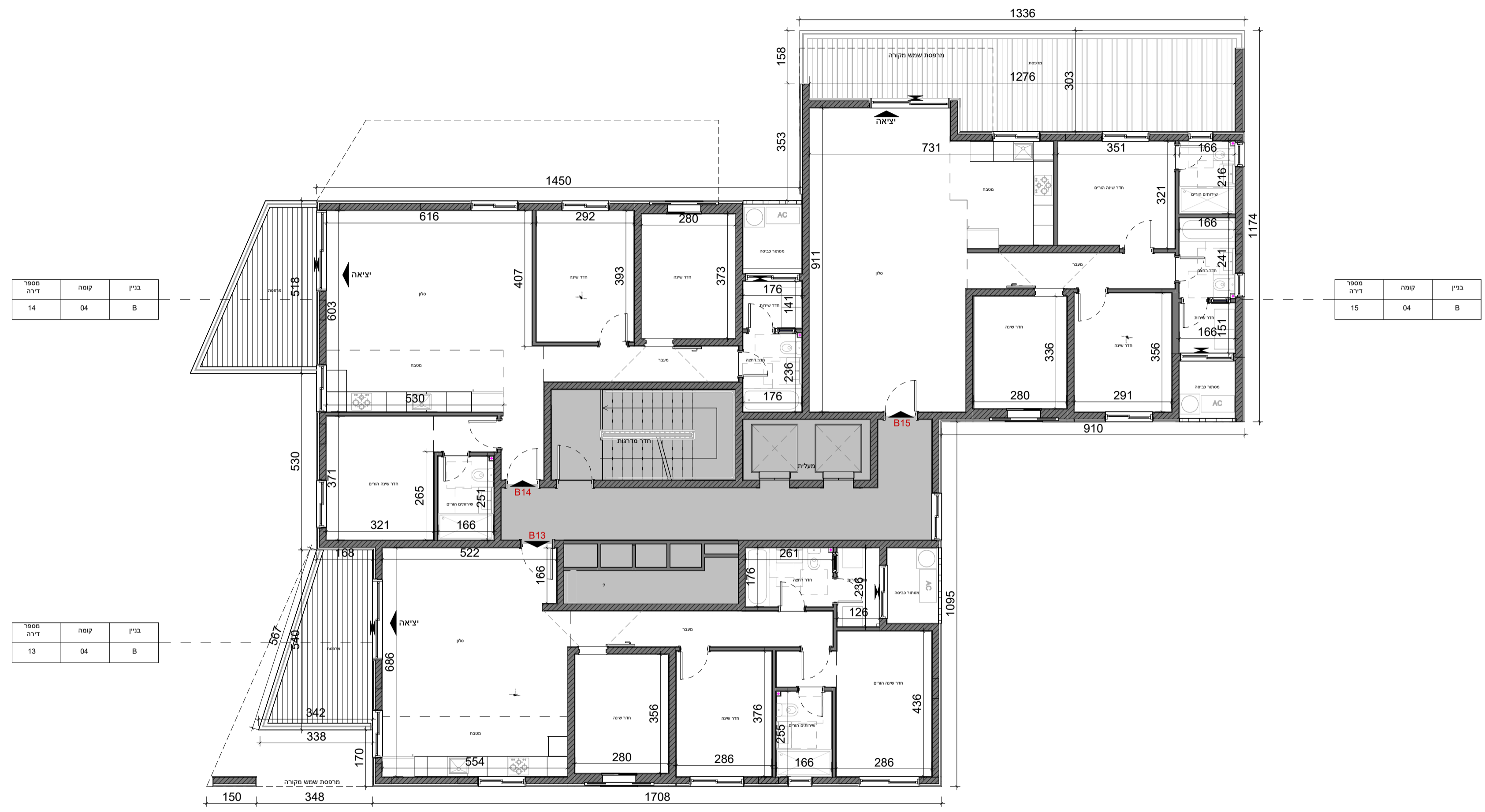
תכנית קומה רביעית 100 : 1קנ"מ
