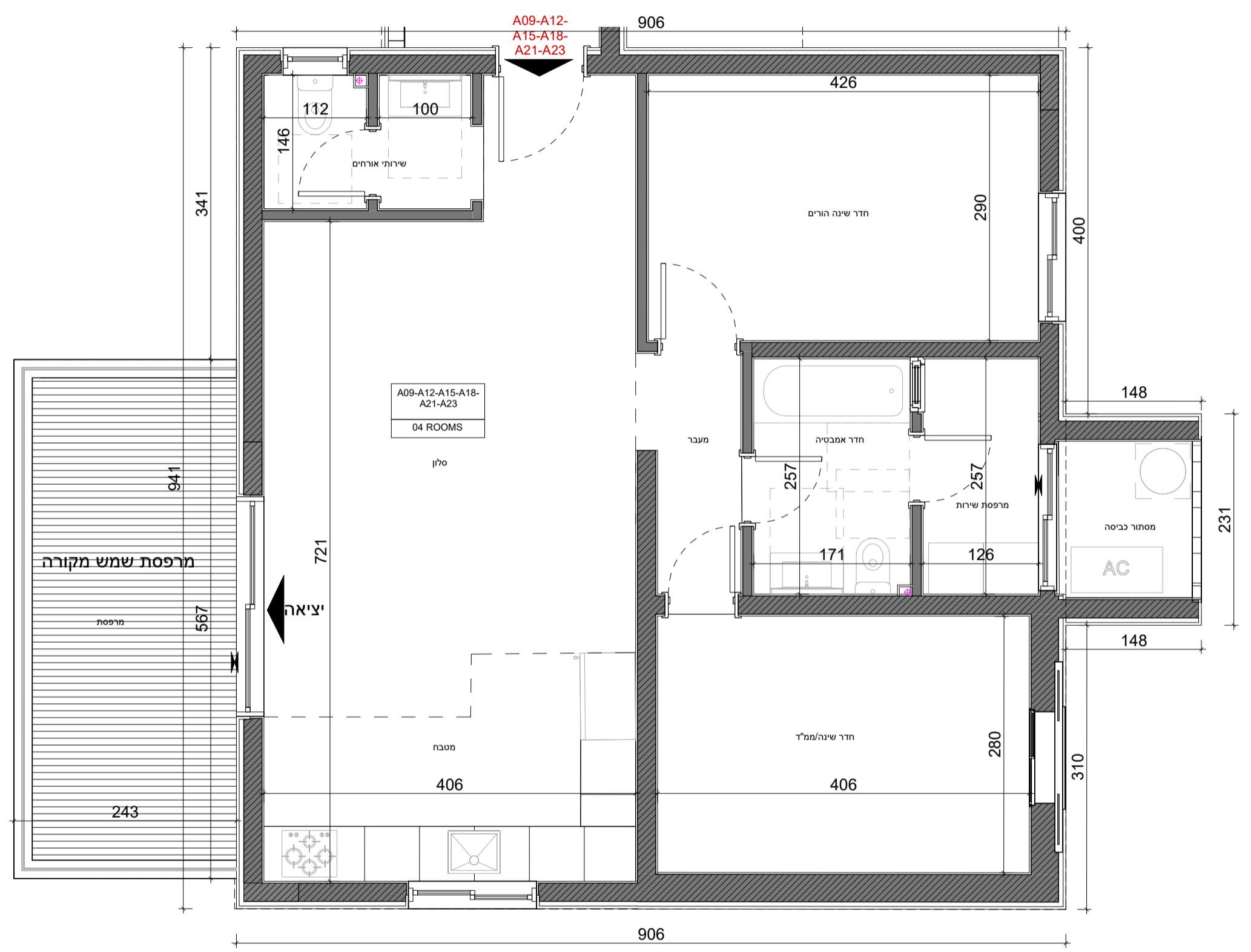
תכנית קומה שנייה 50 : 1 קנ"מ
