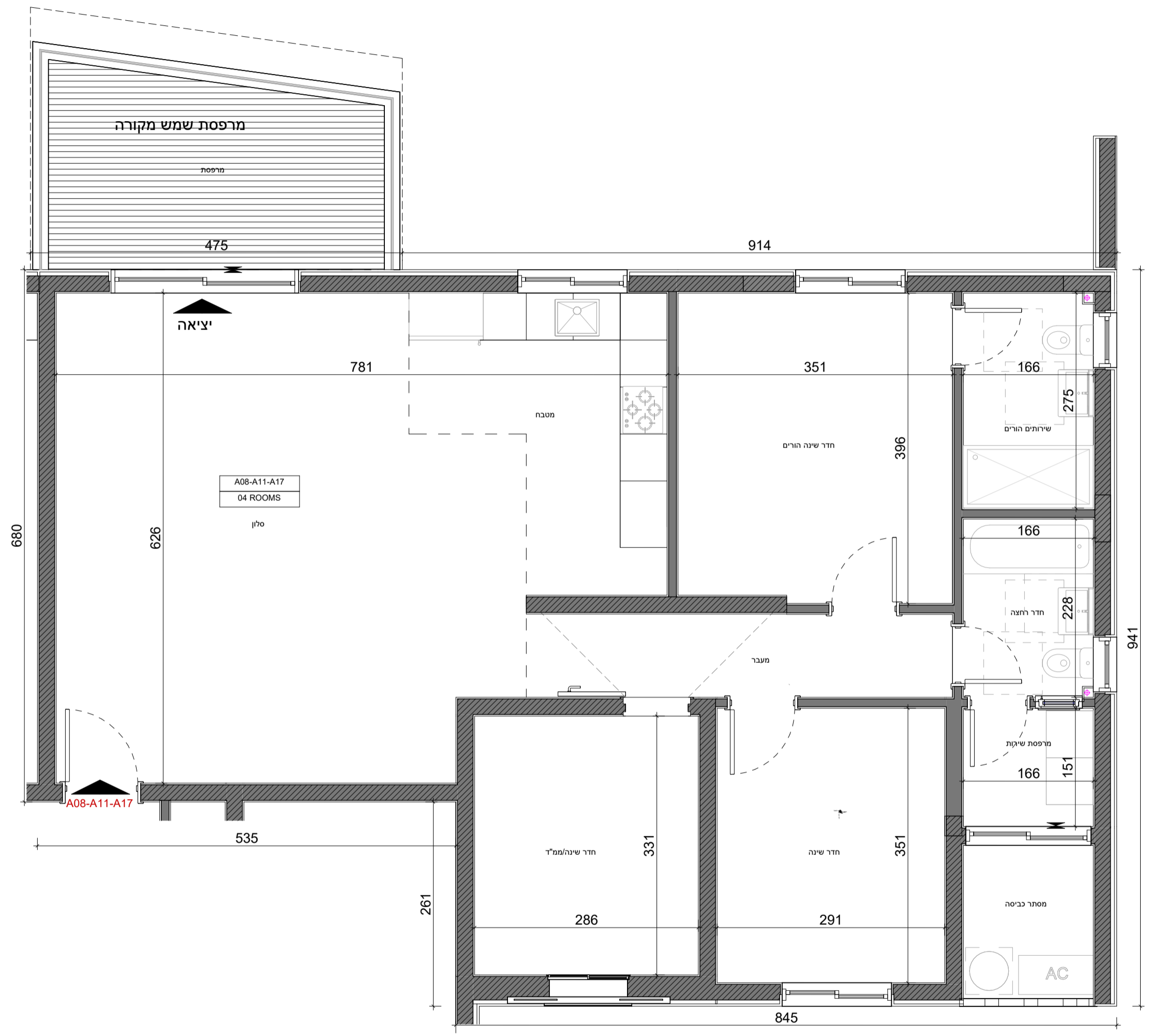
תכנית קומה שנייה 1:50 קנ"מ
